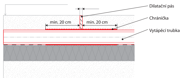
Obr. č. 8: Ochrana vytápěcí trubky při přechodu dilatačním pásem FV PE chráníčkou
